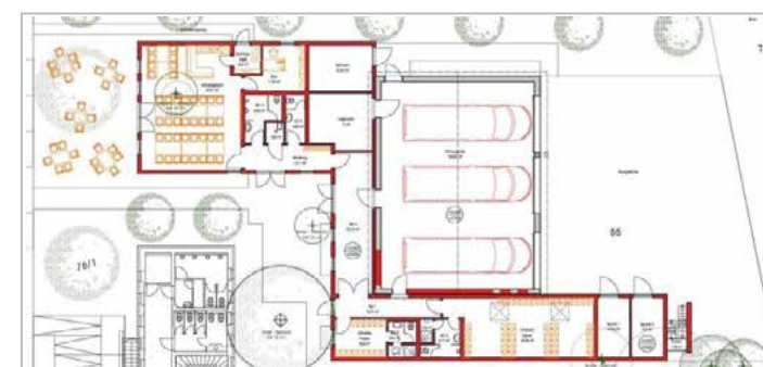
Farbig umrandet der Grundriss des neuen Feuerwehrhauses mit (von oben links im Uhrzeigersinn) Freisitzfläche, Schulungsraum, Fahrzeuggaragen, Garderobe/Technikräume. Am rechten Bildrand die Teplitzer Straße Plan: Architekt Rainer Eis
